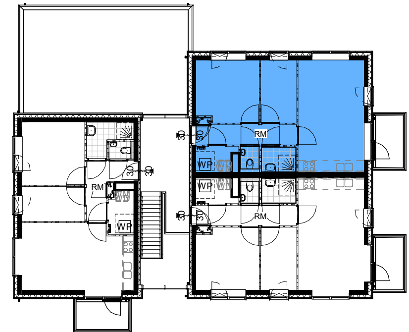
eerste verdieping
