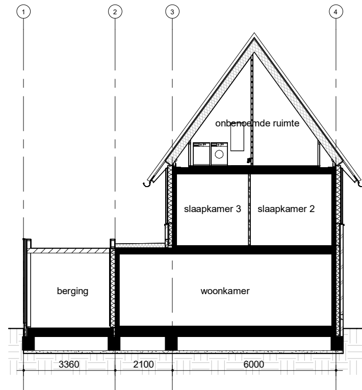
Doorsnede B
