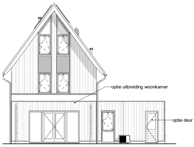
Opties achtergevel
