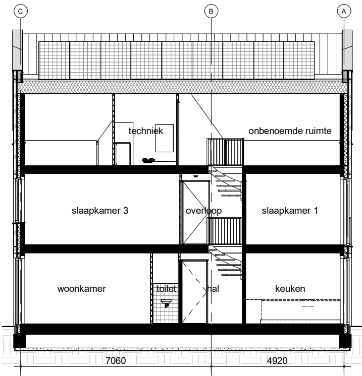
Doorsnede A
