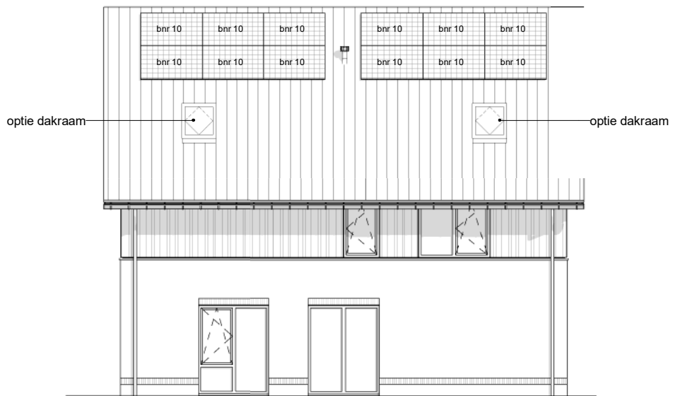
Opties rechtergevel
