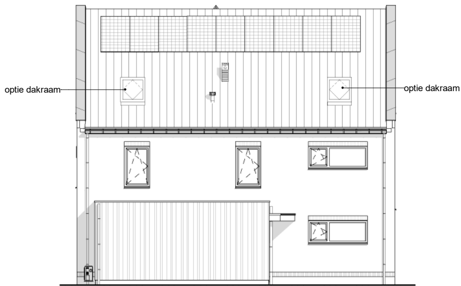
Opties linkergevel
