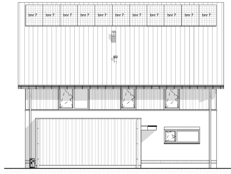
linkergevel
