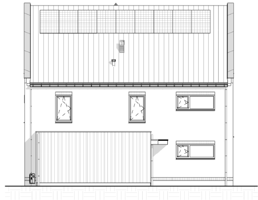
linkergevel
