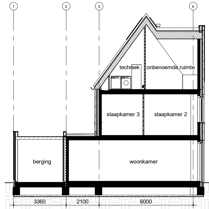
Doorsnede B
