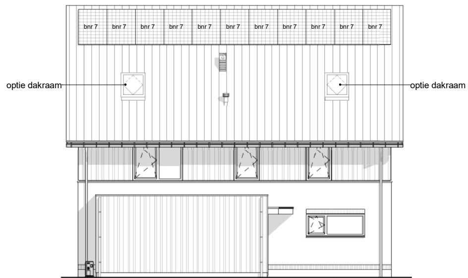
Opties linkergevel
