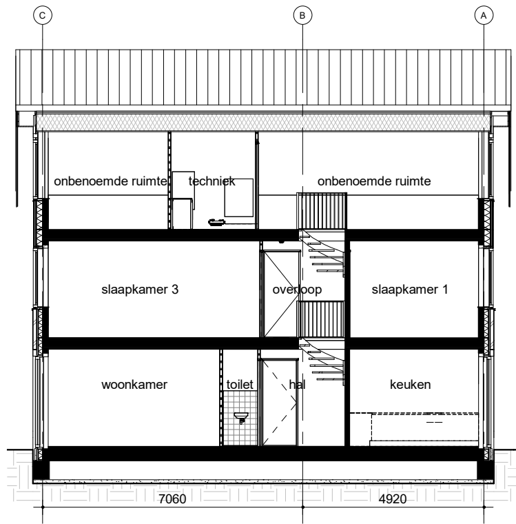
Doorsnede A
