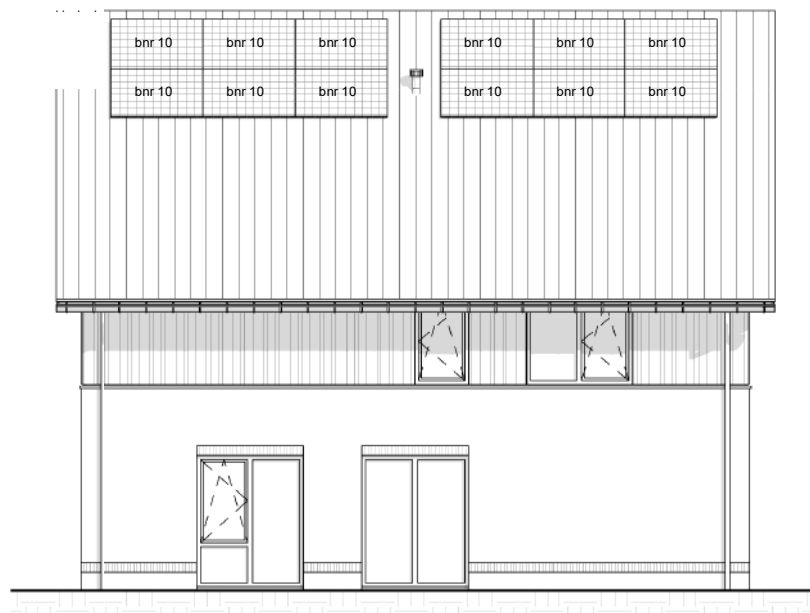
rechtergevel
