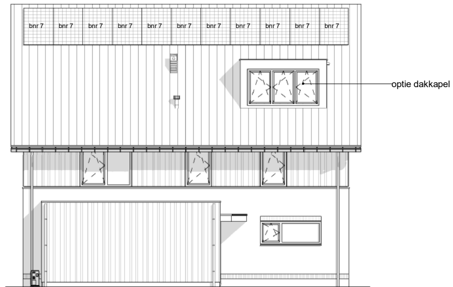
Opties linkergevel
