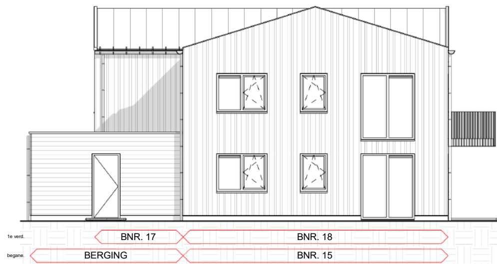
linkergevel
