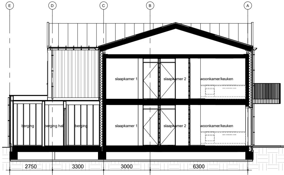
Doorsnede A
