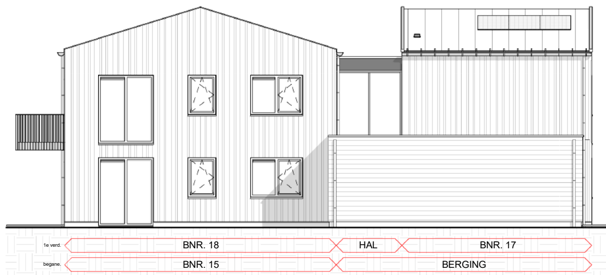
achtergevel
