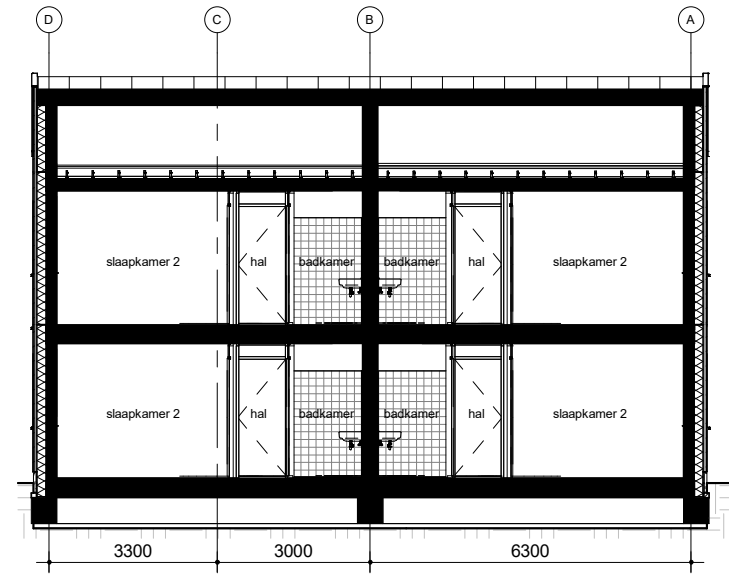
Doorsnede B
