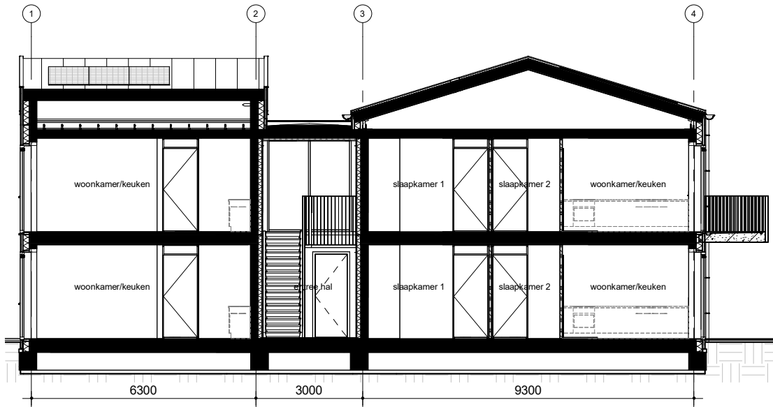
Doorsnede C
