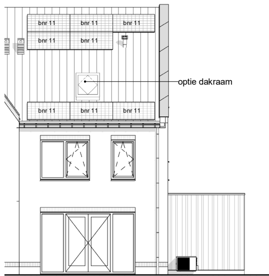
Opties achtergevel
