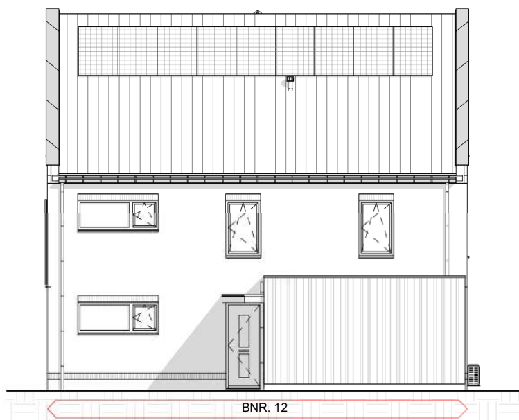
rechtergevel bnr. 12
