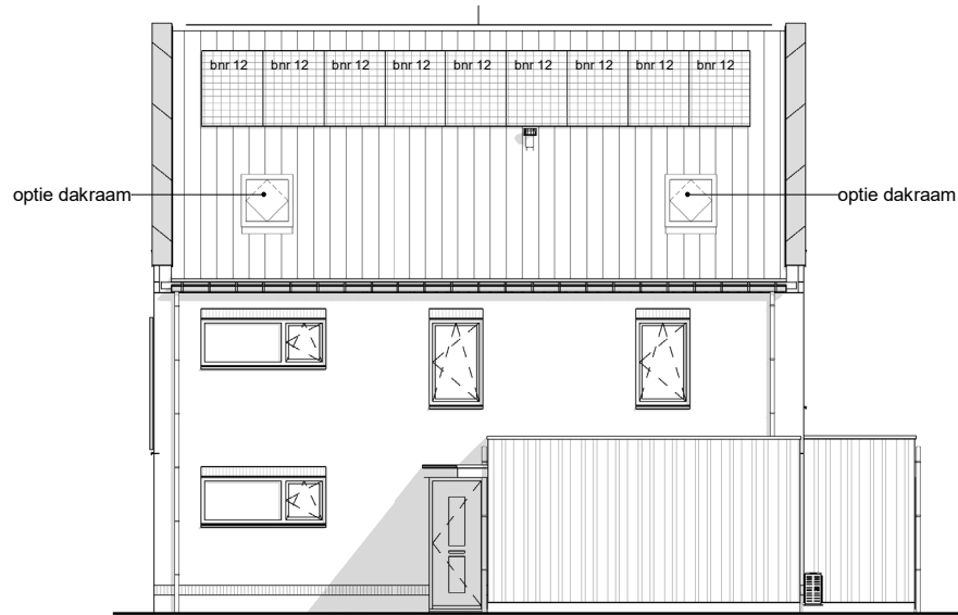
Opties rechtergevel
