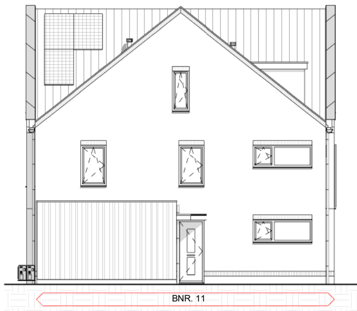
linkergevel bnr. 11
