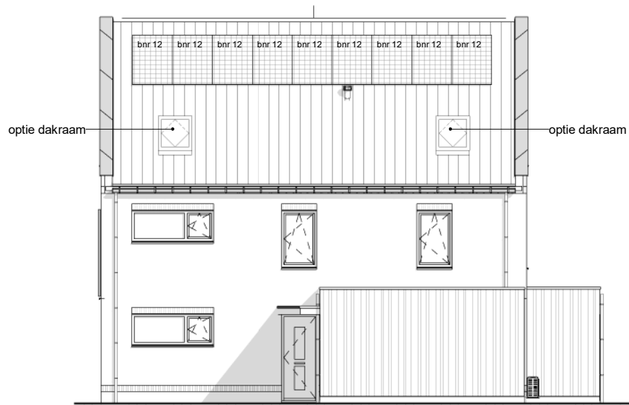
Opties rechtergevel
