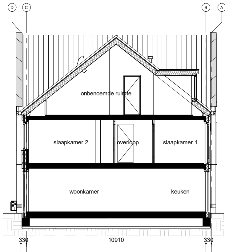
Doorsnede A
