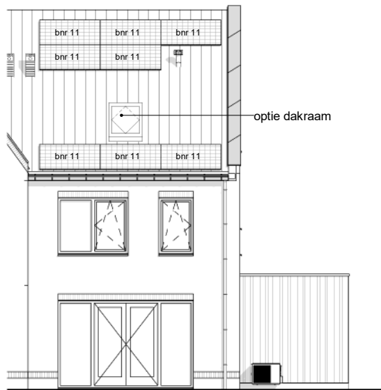
Opties achtergevel
