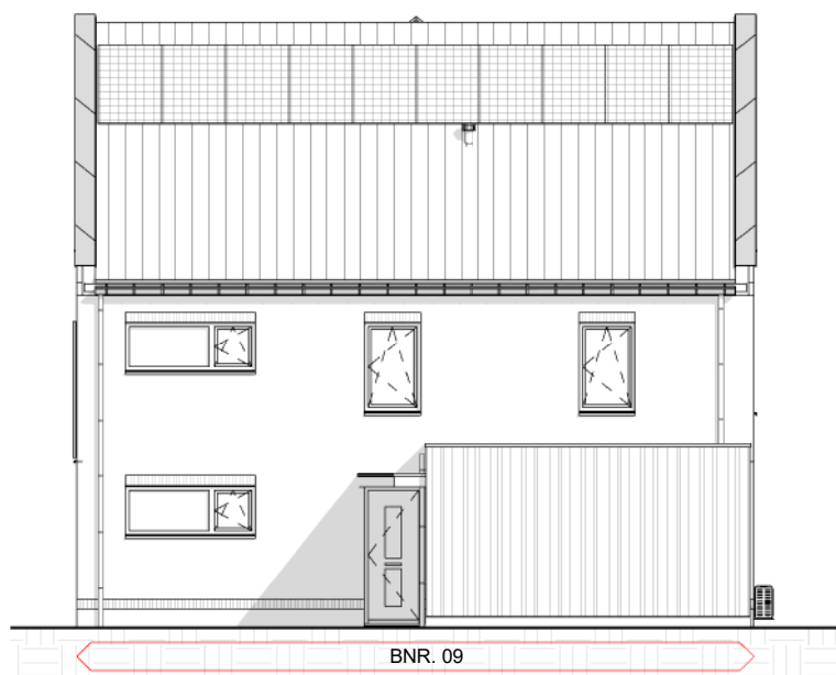
rechtergevel bnr 9
