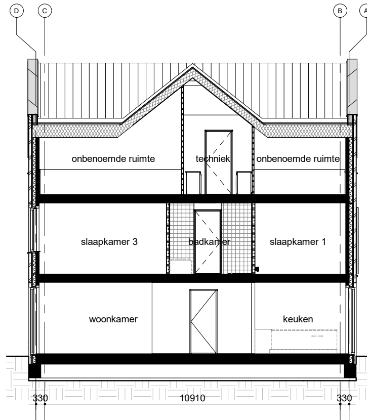
Doorsnede B
