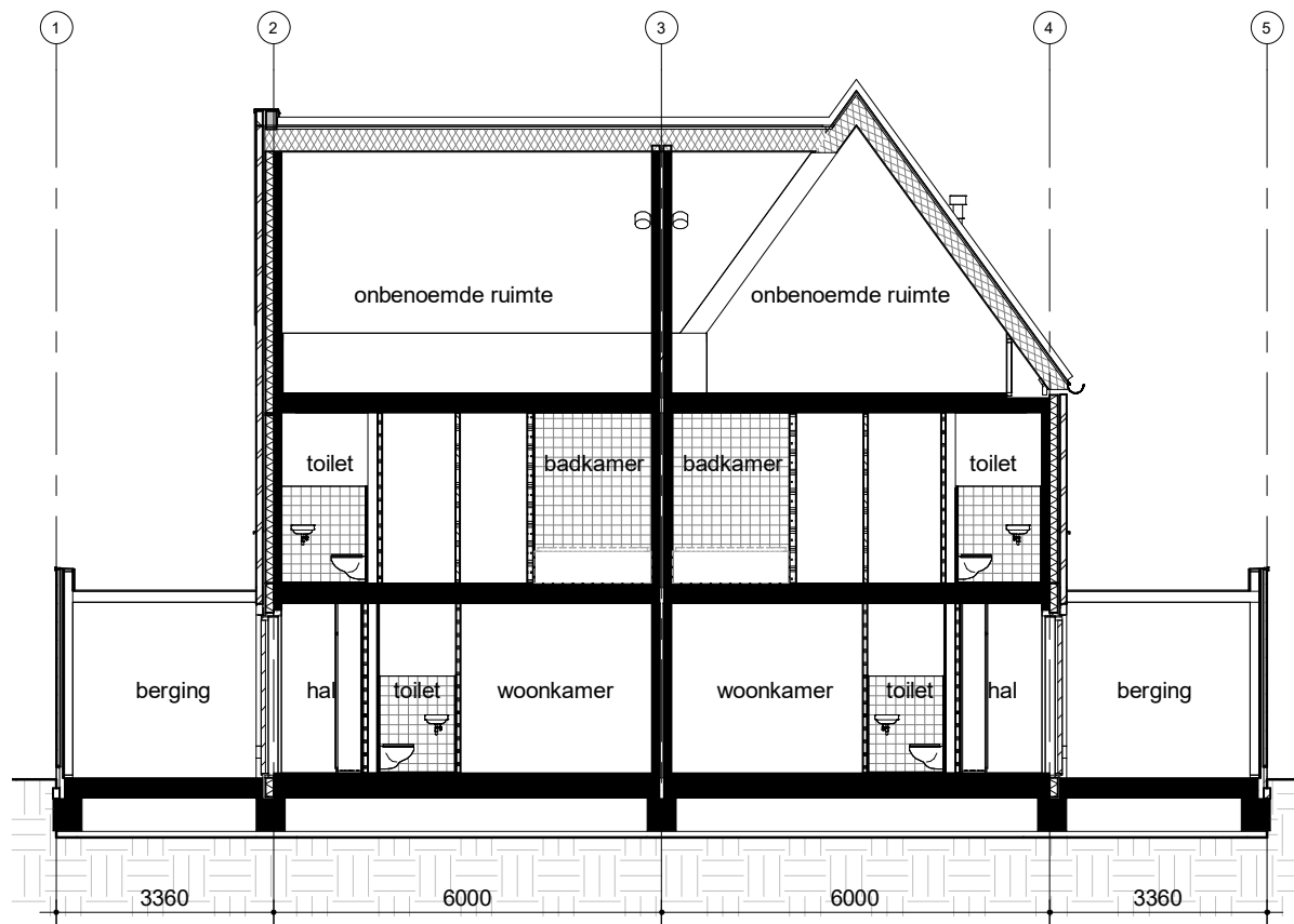
Doorsnede C
